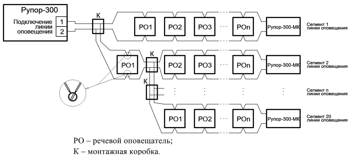
Рисунок 2.2.8. Подключение громкоговорителей к линиям оповещения
